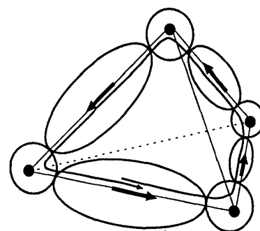
図 5: ヘテロクリニックサイクル近傍の軌道と flow の分解
