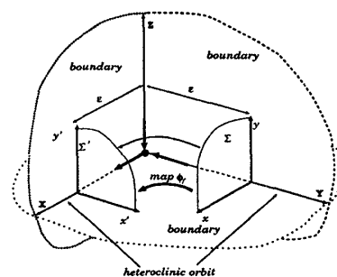
(21) 図 6: 固定点近傍の flow とマップ
