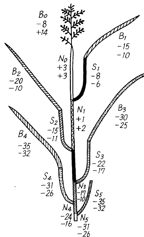
第 2 図 諸器官の伸長と乾物重増加経過の模式図 (B.M.: off season, 品種 Pe Bi Fun) (注) 数字は出穂前後日数 上段 伸長最盛期 下段 乾物増加最盛期
