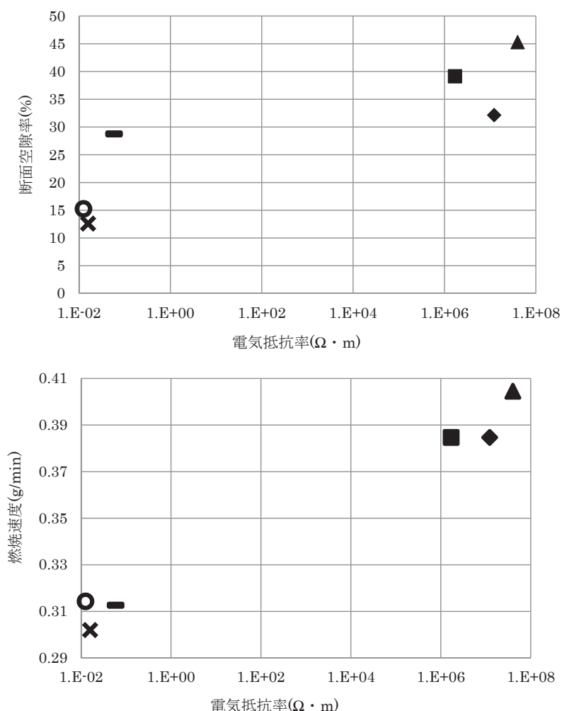
図5 電気抵抗率と断面空隙率（上）や燃焼速度（下）との関係
