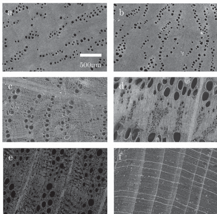
図3 木炭の木口面のSEM画像
