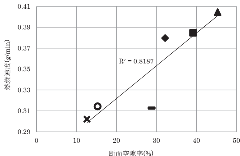
図6 断面空隙率と燃焼速度との関係 プロットは図2参照. ※切炭は測定限界である 4 \times 10^7 \Omega \cdot m の位置にプロットした. Figure 6. Relationship between void ratio of crosscut section and combustion speed.
