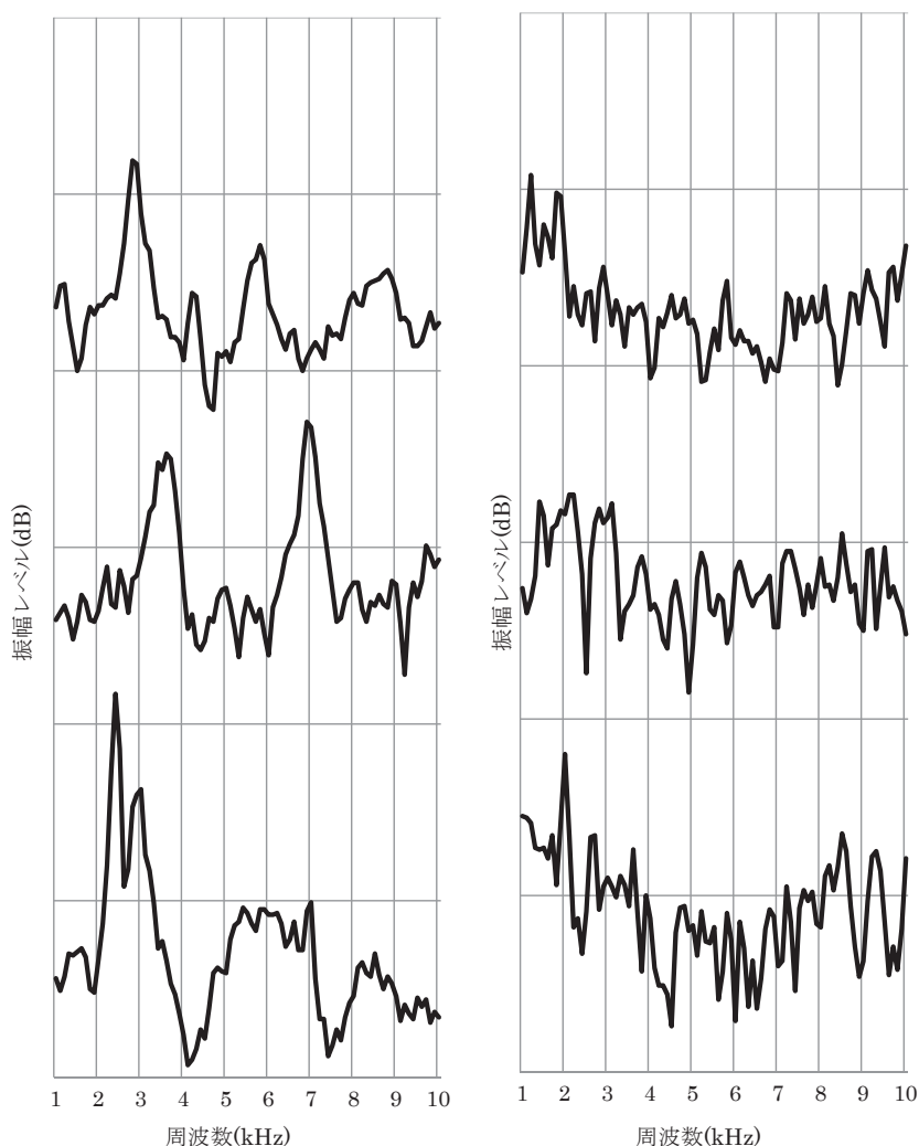
図7 弾性波の周波数スペクトル 左：紀州備長炭，右：土佐黒炭，縦軸は1目盛10dB Figure 7. Frequency spectra of elastic waves propagating in charcoal.
