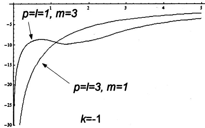
図 3: 近似の誤差 (1)
