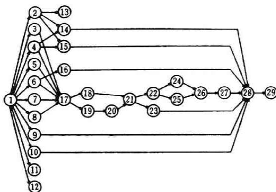
Fig. 1.9. Precedence diagram.
