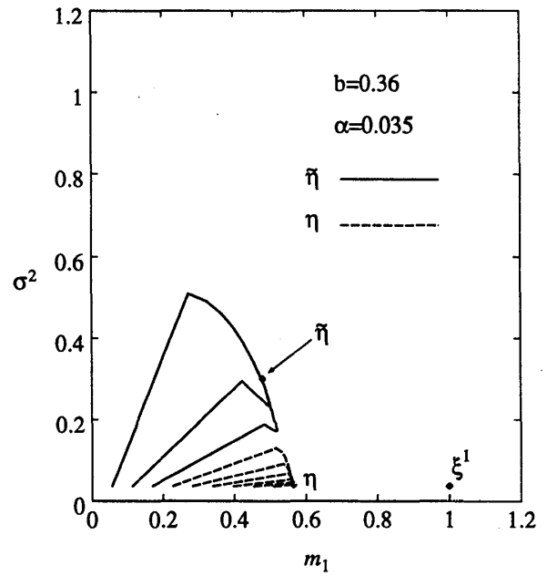
図 4: 一組の相関パターンと \alpha N 個のランダムパターンを覚えさせたモデルの想起過程. 初期状態は P[x_i^0 = \pm 1] = (1 + \eta_i^1 m_0)/2 で与えた.
