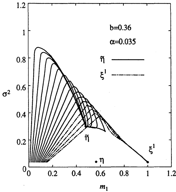
図 3: 一組の相関パターンと \alpha N 個のランダムパターンを覚えさせたモデルの想起過程. 初期状態は P[x_i^0 = \pm 1] = (1 + \xi_i^{1,1} m_0^1)/2 で与えた.
