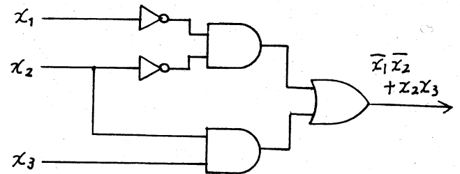
図11 の例題回路C 例：回路C
