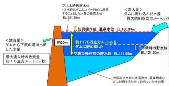
図5 寺内ダム洪水調節の模式図（水資源機構） 3
