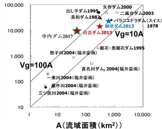
図6 流域面積と流木量の関係 9)
