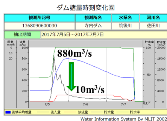
図4 寺内ダム洪水調節（国交省データに加筆）
