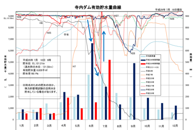
図3 寺内ダム貯水容量変化（水資源機構データに加筆） 2
