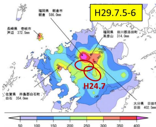
図 1 H29 九州北部豪雨の降雨強度と H24 九州北部豪雨の雨域（500mm 以上）の比較（気象庁データに加筆） 1)
