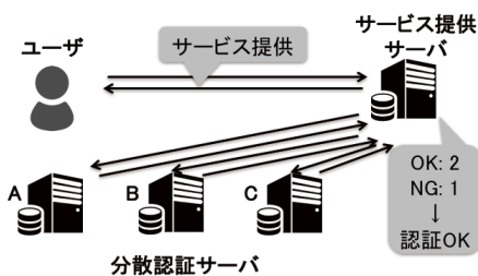
図2 閾値型認証
