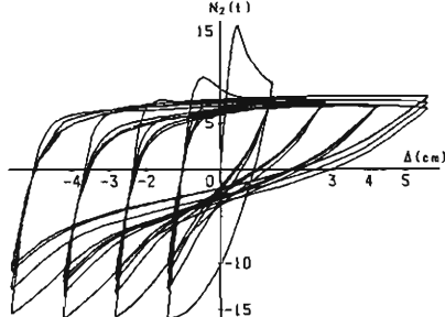
(d) Axial Force in Column ②.
