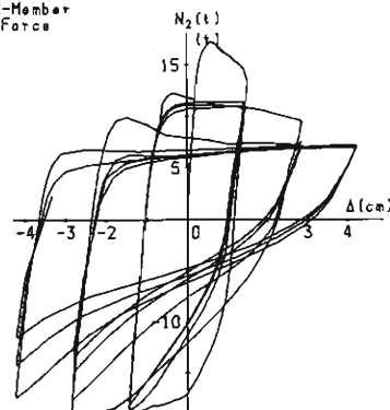
(d) Axial Force in Column ②.
