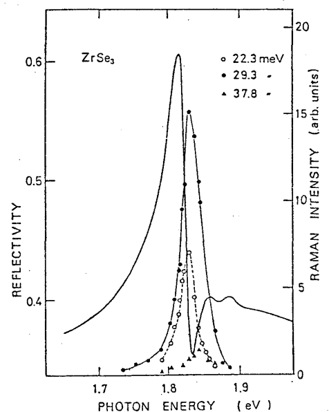
図3 2Kでの反射スペクトルとラマンの励起スペクトル
