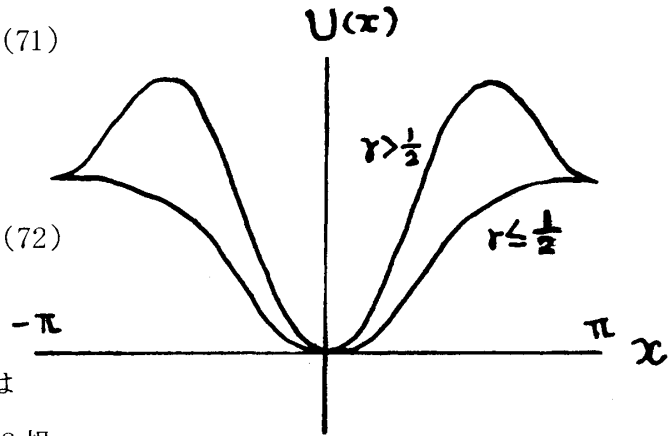
図 7 [III] の振動子のポテンシャル
