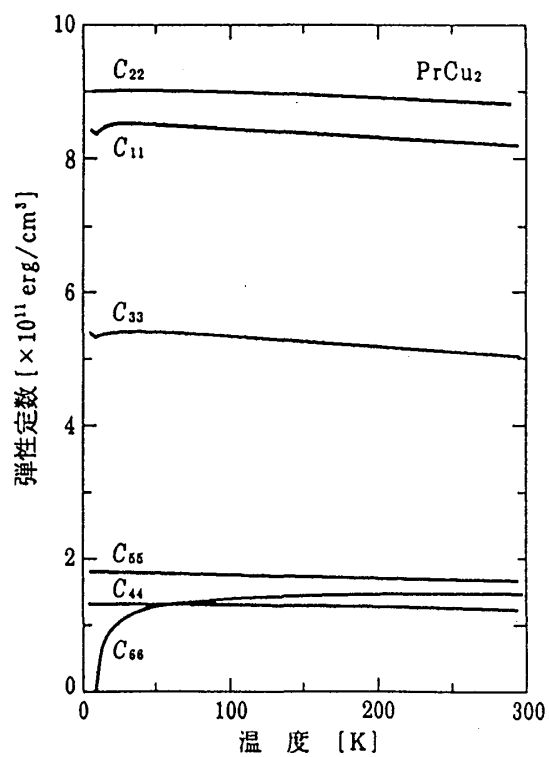
図3.4 \text{PrCu}_2 の弾性定数の温度依存性
