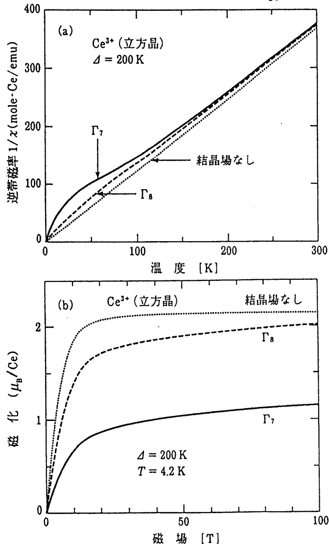
図2.2 立方晶の結晶場効果による \text{Ce}^{3+} イオンの (a) 逆磁化率の温度依存性と (b) 磁化曲線. 点線は結晶場効果を考えない場合であり, 破線は \Gamma_8 が, 実線は \Gamma_7 が基底状態の場合に対応する.
