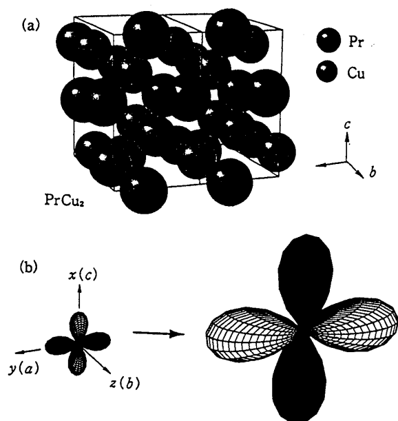
図3.2 (a) \text{PrCu}_2 の結晶構造と (b) 四極子演算子 O_z^2 のメタ磁性に伴う回転.
