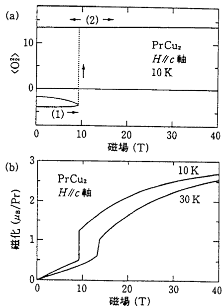
\text{PrCu}_2 のメタ磁性における (a) \langle O_2^2 \rangle と (b) 磁化の磁場依存性.
