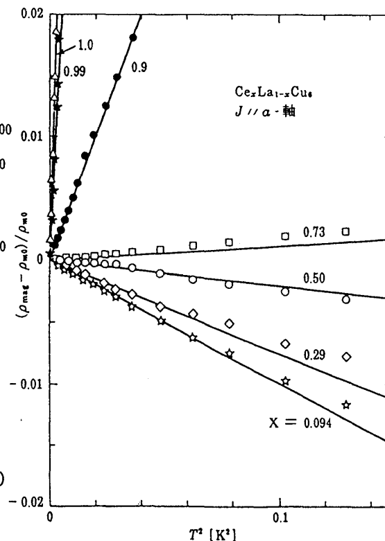
図6.4 Ce x La 1-x Cu 6 の規格化された抵抗の T^2 依存性 (A. Sumiyama, et al. : J. Phys. Soc. Jpn. 55 (1986) 1294.)
