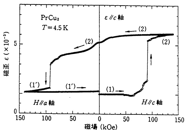
図3.7 磁歪による \text{PrCu}_2 のメタ磁性.
