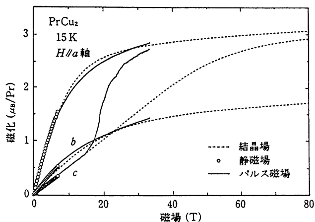
図3.6 \text{PrCu}_2 の磁化曲線. 破線は結晶場とゼーマン効果に基づく理論曲線である.
