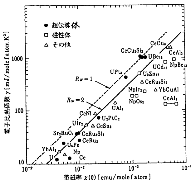
図5.4 T=0 での磁化率 \chi(T=0) と電子比熱係数 \gamma の関係 (P. A. Lee, et al. : Comments on Condensed Matter Physics (1986) Vol. XII.および藤田敏三氏による)
