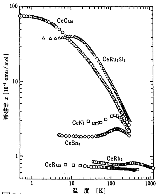
図5.2 磁気秩序を持たない Ce 化合物の帯磁率の温度依存性。
