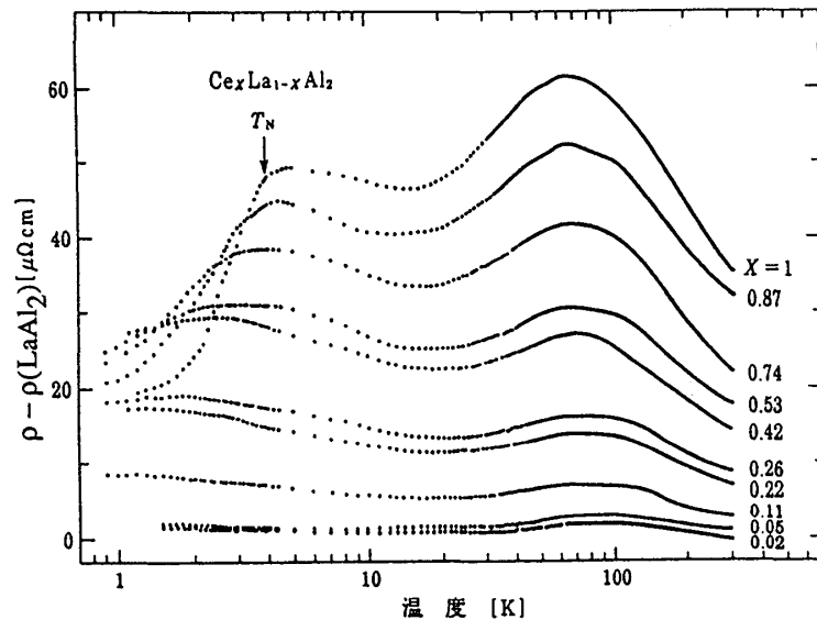
図5.1 \text{Ce}_x\text{La}_{1-x}\text{Al}_2 の磁気的な電気抵抗の温度依存性 (Y. Onuki, et al. : J. Phys. Soc. Jpn. 53 (1984) 2734.)
