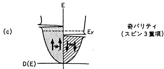
図 9.3 磁場を印加したときの向上きスピンと下向きスピンの状態密度. (a) 常伝導状態ではパウリ常磁性, (b) 超伝導の偶パリティ, (c) 奇パリティでの状態密度
