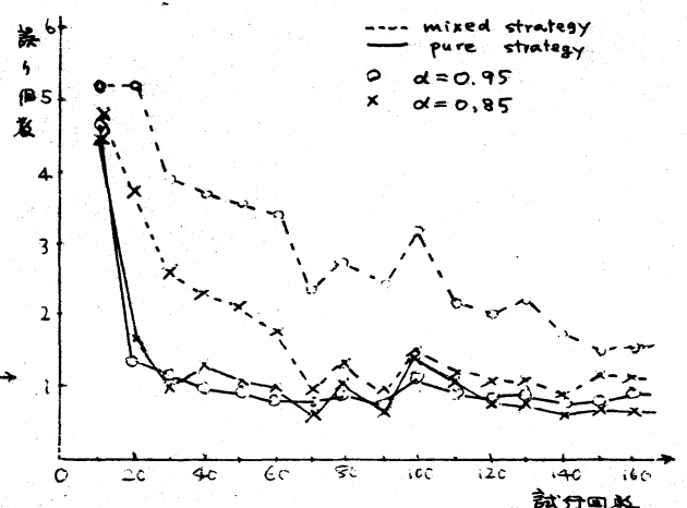
Fig. 5. 誤り回数の変化
