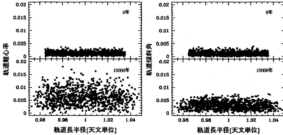
図 2: 初期状態と 1 万年後の粒子の軌道長半径-軌道離心率 (左) と軌道長半径-軌道傾斜角 (右) 上での分布。
