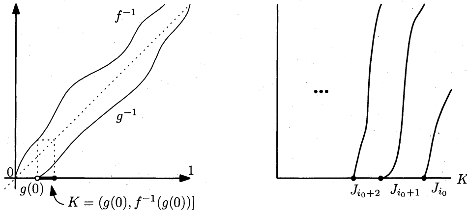
図 1: 区間 K と写像 H の定義の説明. 左図: K の定義の説明. 右図: H のグラフの説明. 各 J_i 上で H = f^{-i} \circ g^{-1} で, i \geq i_0 + 1 のとき H|_{J_i} は J_i から K への微分同相写像となる. 左端点に \{J_i\} が集積しており, よって左側に H の分枝が集積している.
