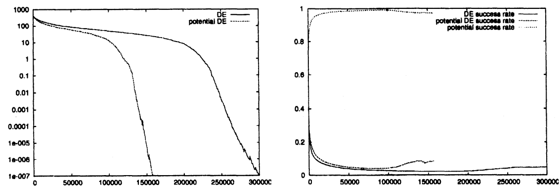
図 5: f_4 における関数値および成功率の変化
