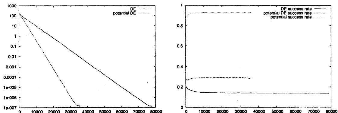
図 2: f_1 における関数値および成功率の変化
