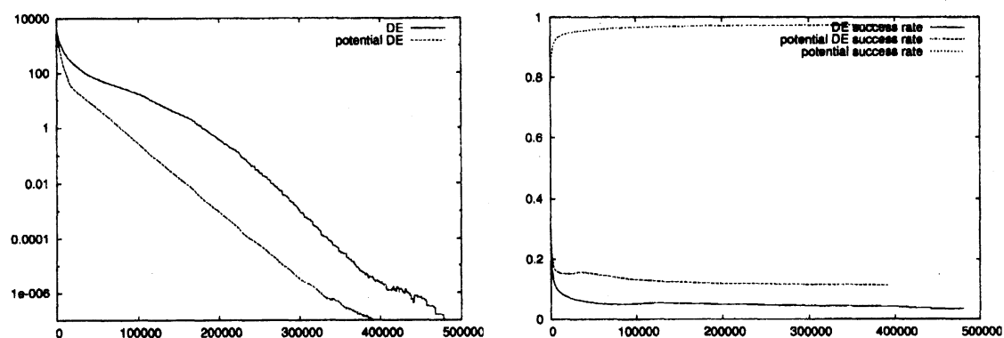
図 3: f_2 における関数値および成功率の変化
