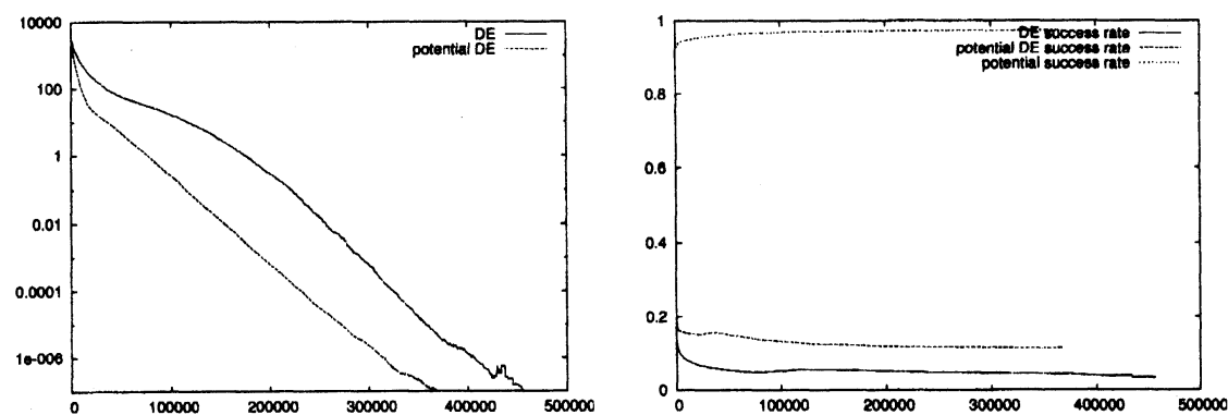
図 4: f_3 における関数値および成功率の変化
