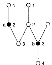
図 1 できるだけレベルが小さくなるようにレベル付けし、レベルを G の彩色とする
