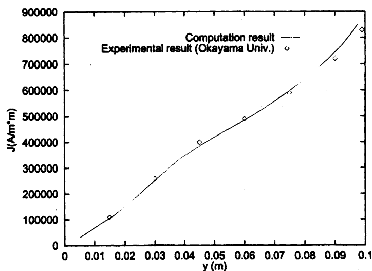
図 5.3: 電気学会渦電流問題結果
