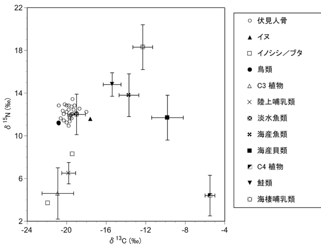
図 1. 伏見城跡遺跡から出土した江戸時代人骨と動物骨，ならびに各食物群の炭素・窒素安定同位体比の比較。各食物群の値は，生体濃縮の値として，炭素同位体に 4.5‰，窒素同位体に 3.4‰を加えて補正した。
