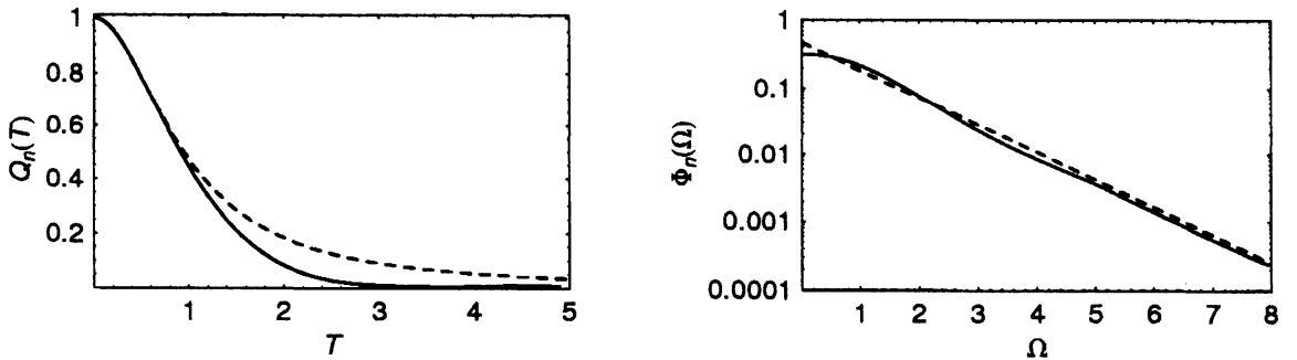
図 3: 左図は相関関数 Q_n(T) で, 実線が KS 方程式の数値計算, 破線が (22) を示す. 右図はパワースペクトル \Phi_n(\Omega) で, 実線が数値計算, 破線が (23) を示す. とともに, k_n = 0.69 の場合であり, \tilde{\tau}_n = 0.44 .
