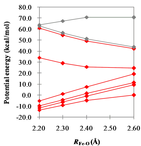
(C) 6SA-CASSCF(9,8)
