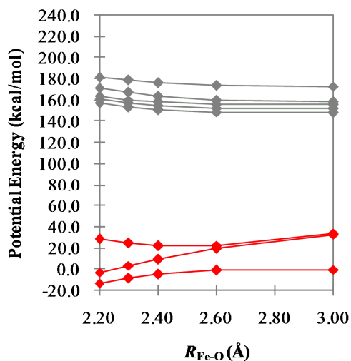
(C) 3SA-CASSCF(9,8)
