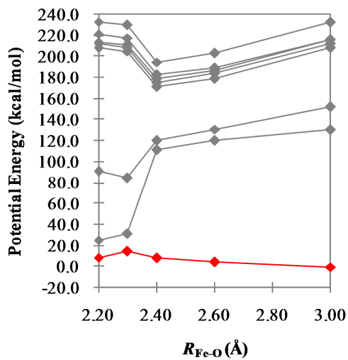
(A) SS-CASSCF(9,8)
