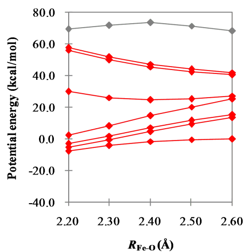
(D) 7SA-CASSCF(9,8)
