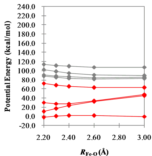
(D) 4SA-CASSCF(9,8)
