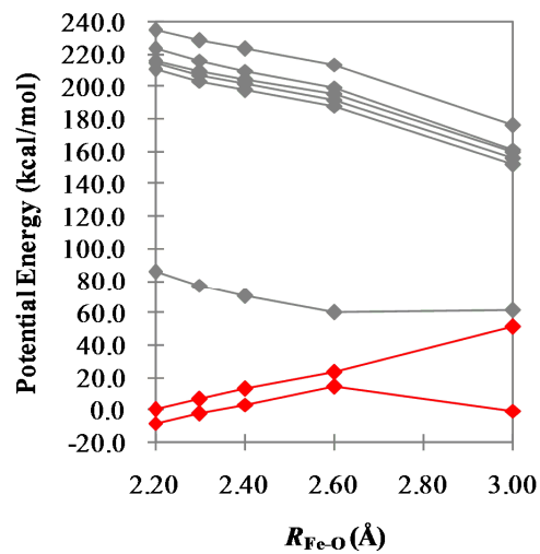
(B) 2SA-CASSCF(9,8)
