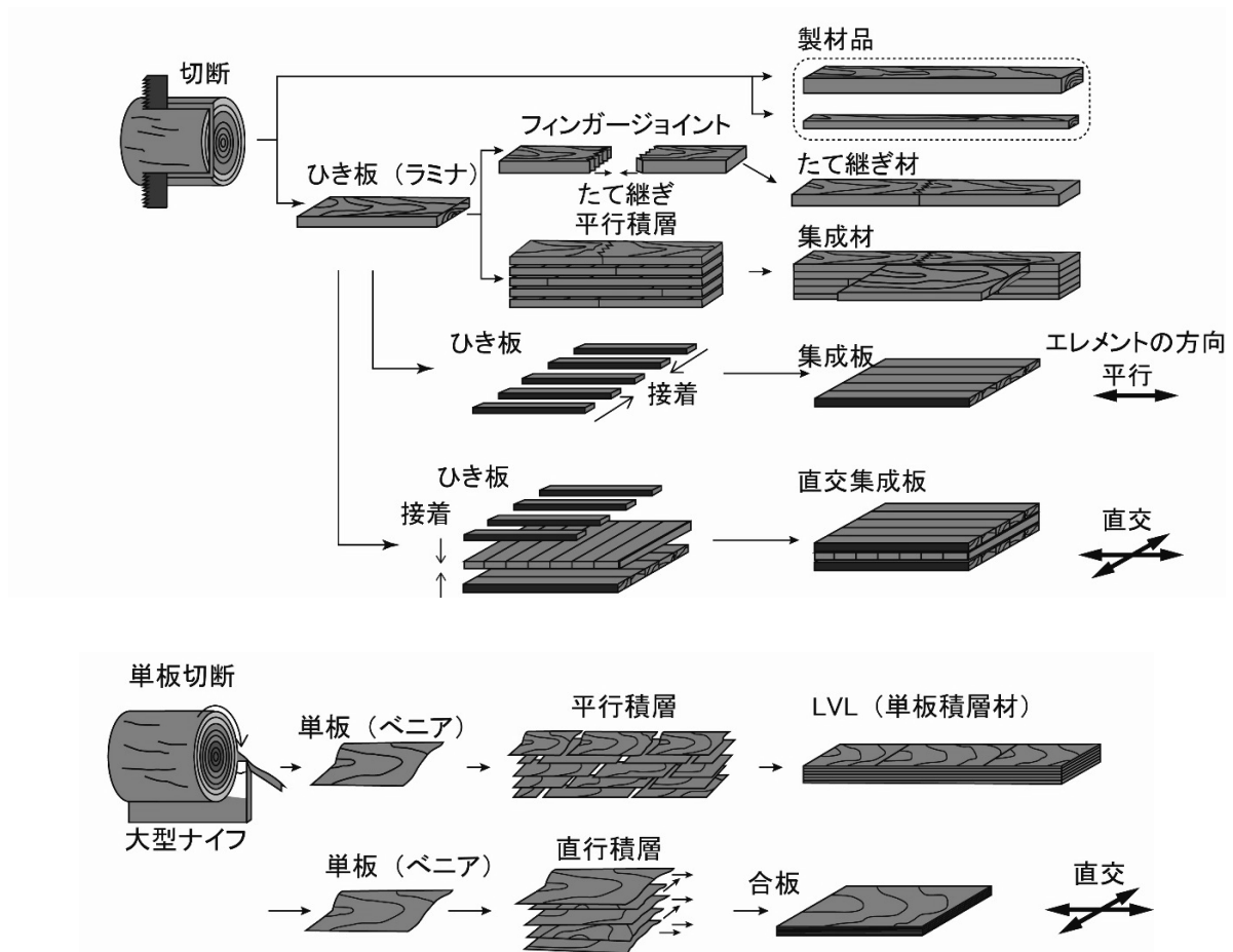
図2 さまざまな木材をベースとする材料 2)
