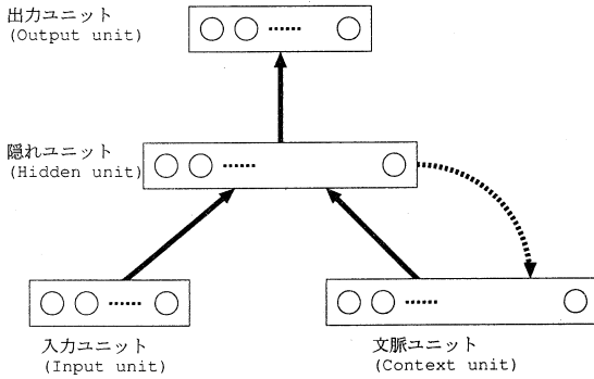
図 1: 単純回帰ネットワーク
