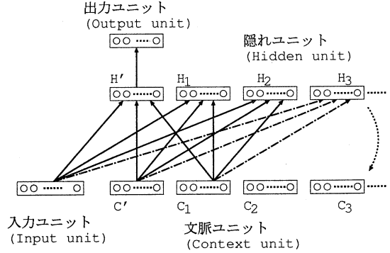
図 2: 拡張単純回帰ネットワーク
