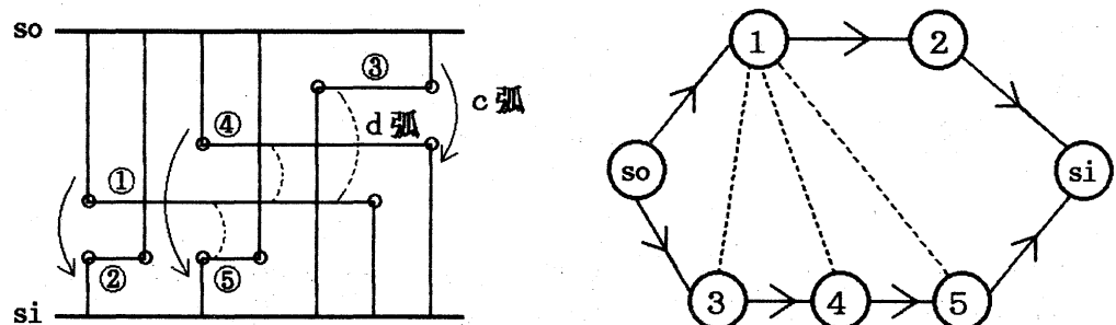
図5. 配線経路決定問題と選択グラフ
