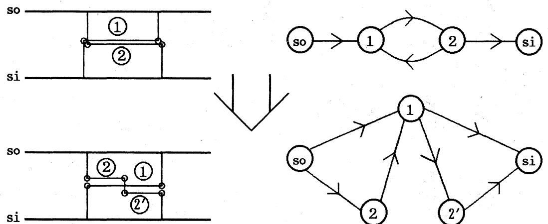
図6. 有向閉路の除去
