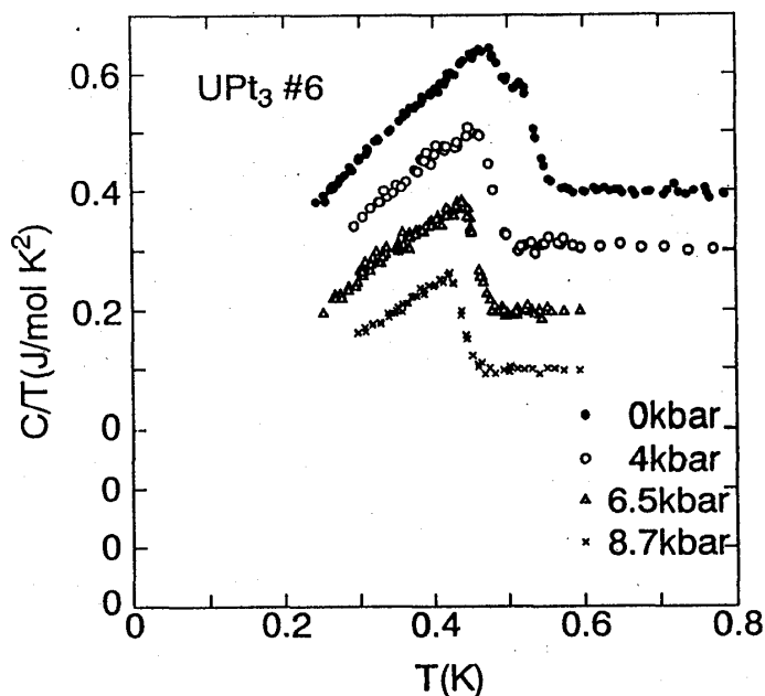
図1 UPt 3 の圧力下比熱 ( C/T-T^2 プット)
