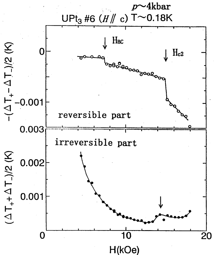
図2 圧力下UPt 3 の磁気熱量効果 実線はアイガイドのため
