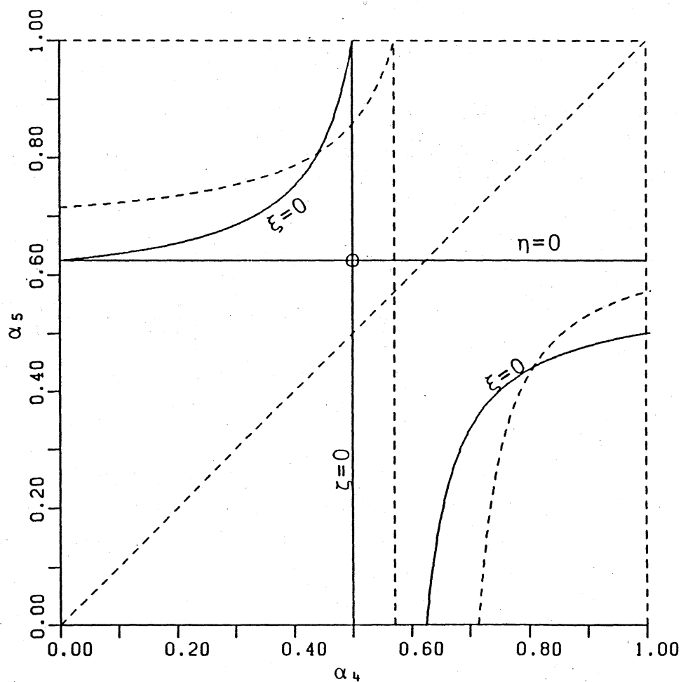
図1 \xi, \eta, \zeta = 0 の曲線 ----- は禁止線, \circ \cdots (\frac{1}{2}, \frac{5}{8})
