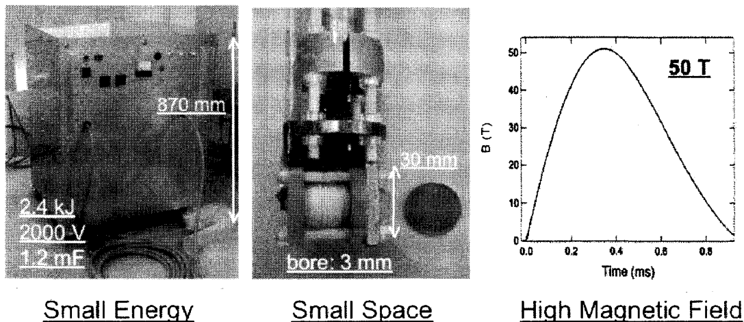
図 11: 超強磁場放射光実験に用いるポータブルパルス磁場システム。
