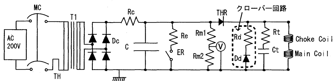
図 2: パルス磁場電源の回路図, 記号に関しては本文参照
