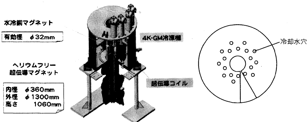
図 1: 金属材料研究所のヘリウムフリー型ハイブリッド磁石と簡単なビッター板の図
