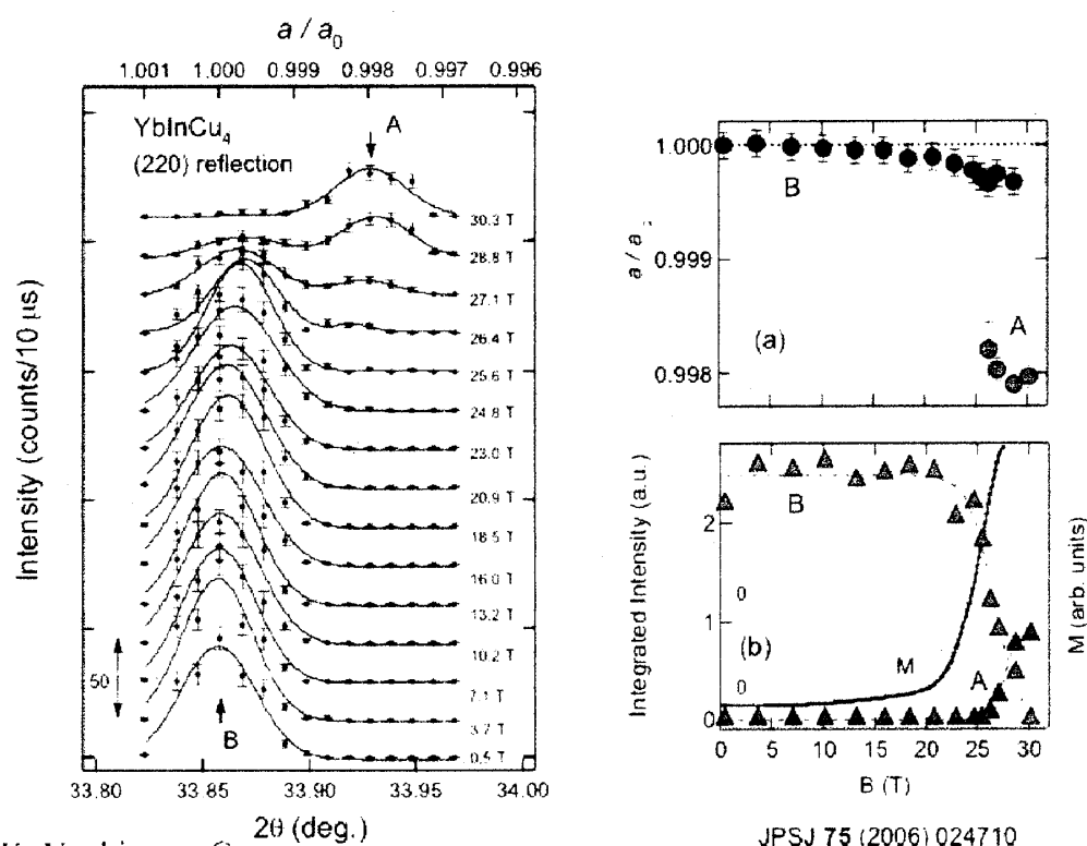
図 12: YbInCu 4 における磁場誘起価数転移における格子定数の磁場変化。
