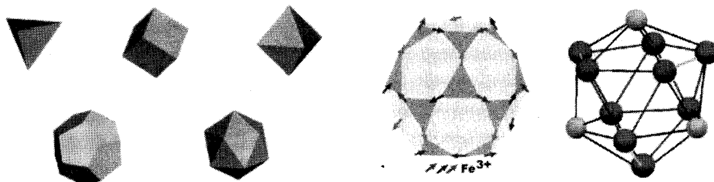
図 7: 5つのプラトン多面体と2つのスピン多面体クラスター。 \text{Mo}_{72}\text{Fe}_{30} は20の三角形と10の五角形からなる Icosidodecahedron と呼ばれる多面体で30の頂点を \text{Fe}^{3+} イオンが占有する。 \text{Fe}_9 は三角からなる Icosihedron と呼ばれる多面体であるが12の頂点のうち9つを \text{Fe}^{3+} イオンが、残りの3つを非磁性のPイオンが占める不完全な多面体である。
