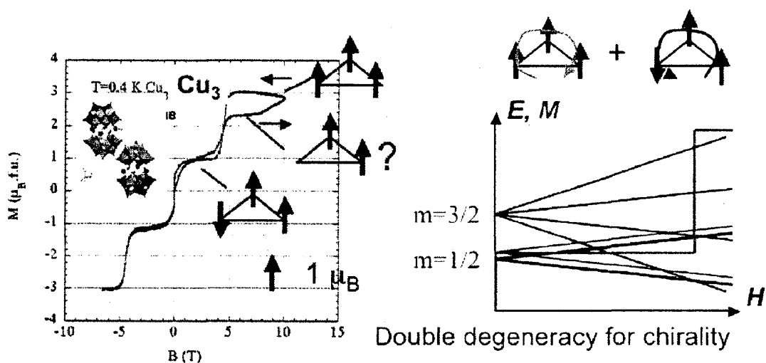
図 8: 3角リングの頂点に S=1/2 の \text{Cu}^{2+} スピンをおいた \text{Cu}_3 の1サイクルのパルス磁場中での磁化過程。矢印は磁場の変化の向きを示す。それぞれの状態のスピン配置を絵で示す。エネルギー準位は右図のようになり、基底状態に2つの2重項が存在する。
