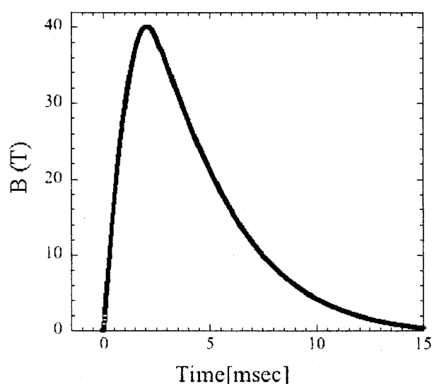
図 3: パルス磁場電発生波形の一例
