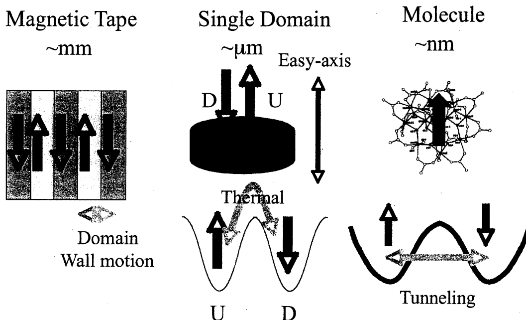
図 5: バルクの強磁性体、微粒子、単分子磁石とそれぞれの磁化反転の機構
