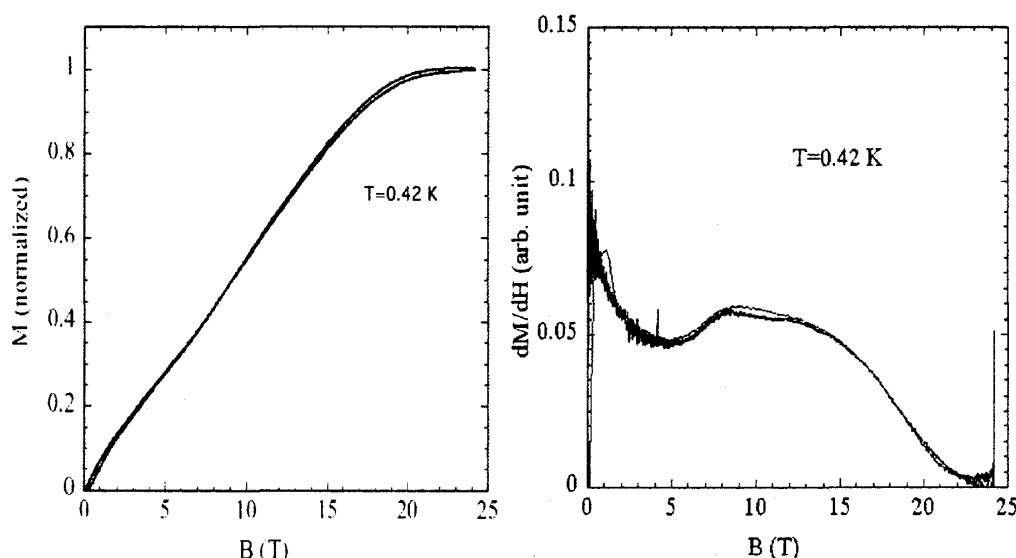
図 9: \text{Mo}_{72}\text{Fe}_{30} の磁化過程。左が磁化曲線、右は磁化の磁場微分を示す。
