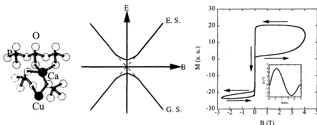
図 10: 磷酸ガラス中にドーピングした S=1/2 の Cu スピンの磁化過程。エネルギー準位は 2 準位のみで表される。
