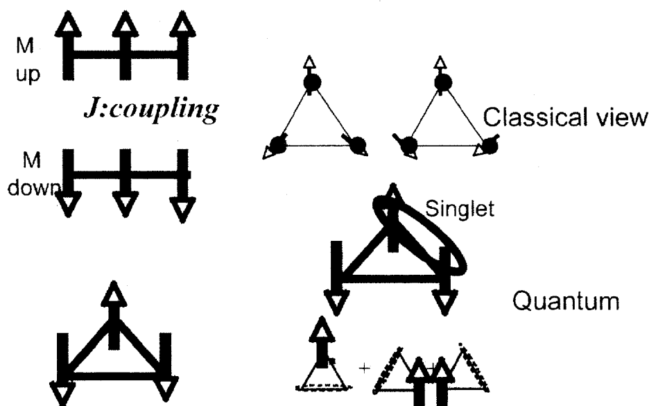
図 6: スピンをリング状にするとスピнкаイラリティが生じる。3 角リングでは古典的な場合は、カイラリティの違いは 2 つの 120 度構造として表される。量子系では、リングとしての波動関数を 3 つの等価な状態から合成するときの波動関数の位相によって定義され、波動関数の対称-反対称に対応する。
