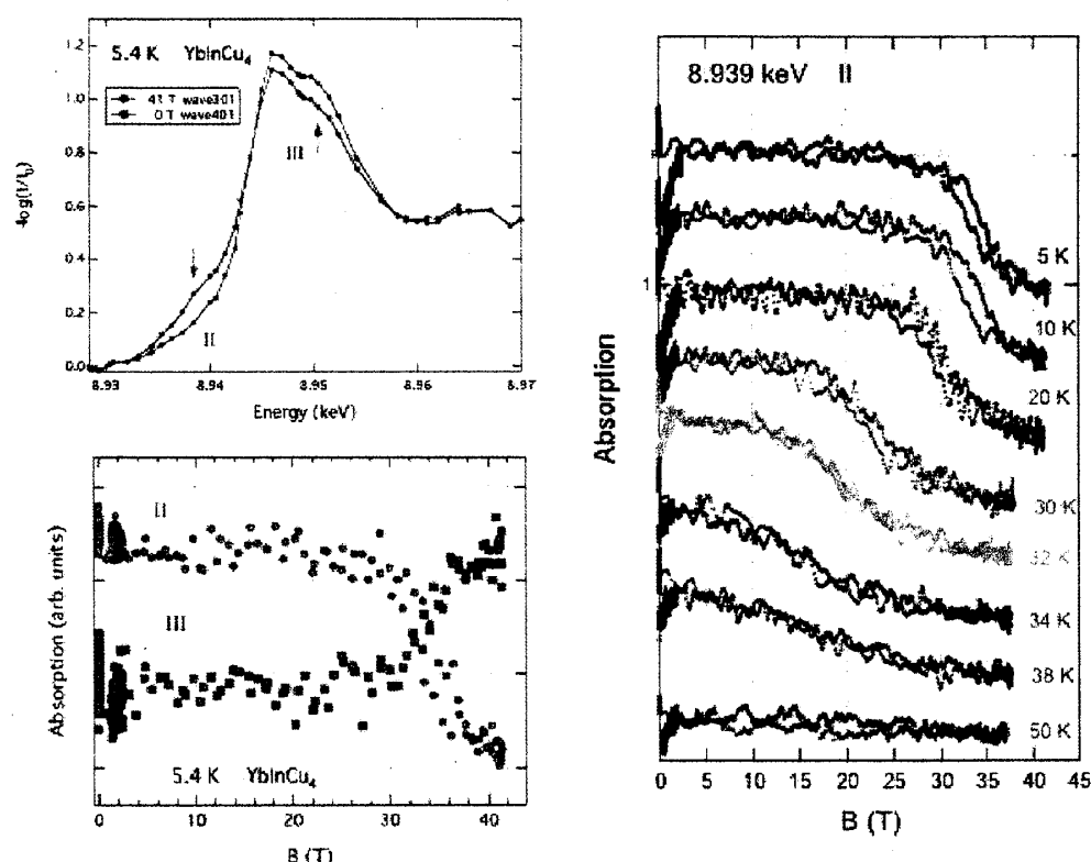
図 13: YbInCu 4 における磁場誘起価数転移における超強磁場 XAS スペクトル。
