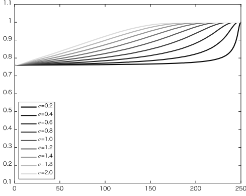
Figure 12: X_T(\omega) = x_1(\sigma を動かした場合)
