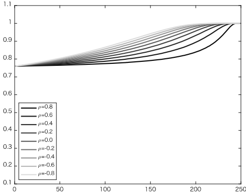
Figure 14: X_T(\omega) = x_1(\rho を動かした場合)
