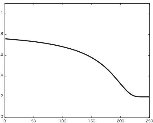
Figure 9: X_T(\omega) = x_0 = 0.2 のベースライン
