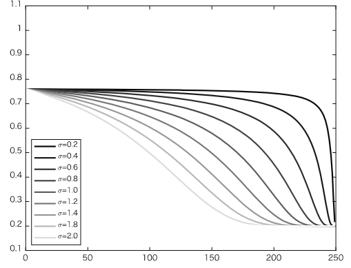
Figure 13: X_T(\omega) = x_0(\sigma を動かした場合)
