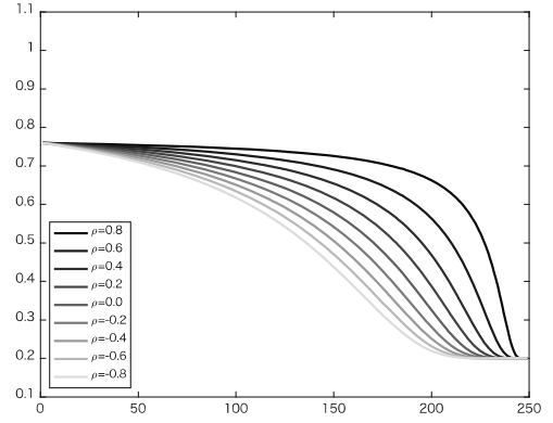
Figure 15: X_T(\omega) = x_0(\rho を動かした場合)
