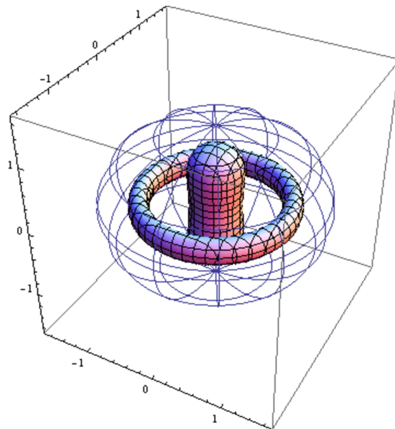
図 14: 扁平回転楕円体内部における Dirichlet 境界条件下でのラプラシアンの固有関数の等高面の一例. 固有値 16.61.
