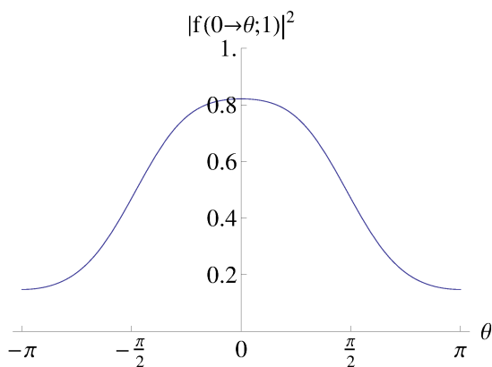
図 3: k^2 = 1 . 入射方向 0.
