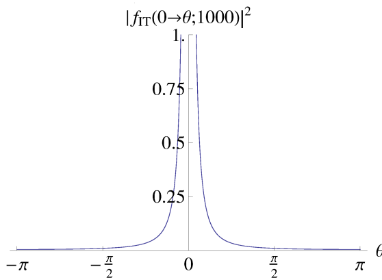
図 11: 伊藤-田村公式. 入射方向 0.
