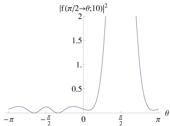
図 6: k^2 = 10 . 入射方向 \pi/2 .
