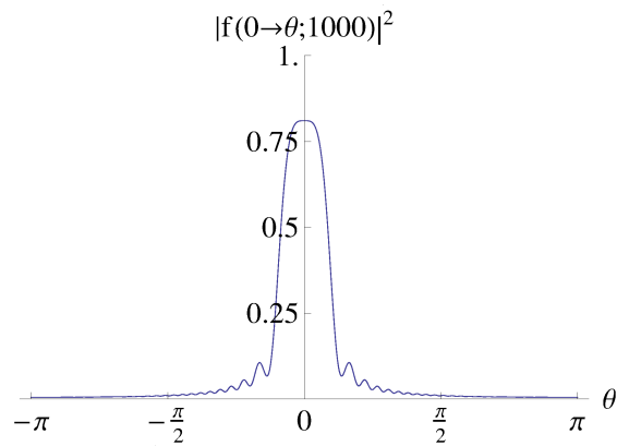
図 12: 我々の結果. 入射方向 0.
