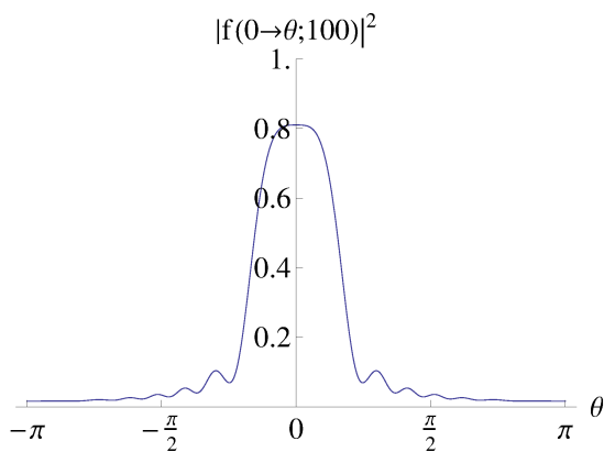
図 7: k^2 = 100 . 入射方向 0.
