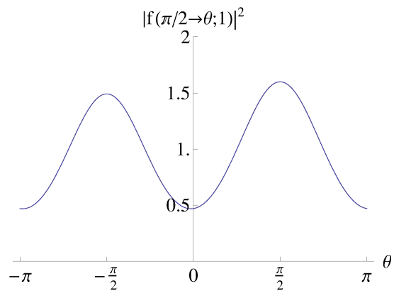
図 4: k^2 = 1 . 入射方向 \pi/2 .
