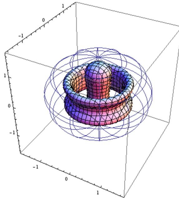
図 16: 扁平回転楕円体内, ディリクレ境界条件下での無限に細い輪状のソレノイド R に閉じ込められた磁場に対する Schrödinger 作用素の固有関数の等高面の一例. 固有値 22.22.
