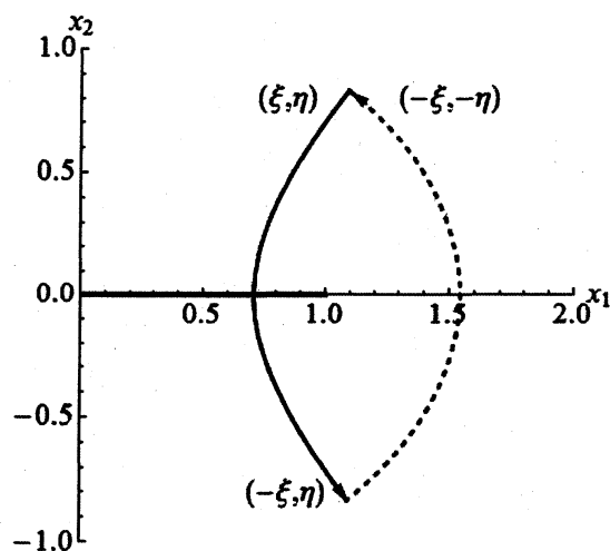
図 2: 楕円座標 (\xi, \eta) の点から出発し, \xi を -\xi まで変えたのち, \eta を -\eta まで変えると元の点に戻る.
