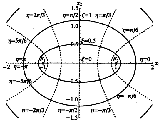
図 1: 楕円座標の座標曲線 ( a = 1 ). \xi = \text{一定} の曲線は楕円または線分, \eta = \text{一定} の曲線は双曲線または半直線となる.
