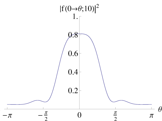
図 5: k^2 = 10 . 入射方向 0.
