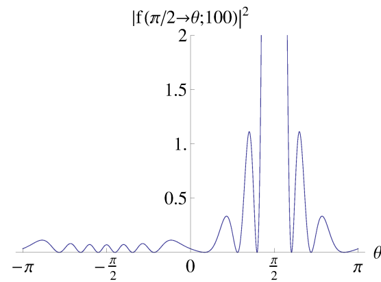
図 8: k^2 = 100 . 入射方向 \pi/2 .
