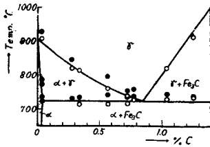
Fig. 7. Section II ( As=0.0\% ).
