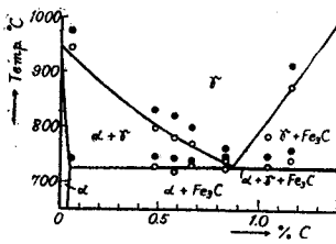
Fig. 9. Section IV ( As=0.5\% ).
