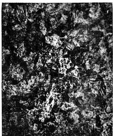
Photo. 3 \times 450 C=0.14%, As=1.09% 986°C. \times 30 min. W.Q. 5% Picral etch. Martensite.
