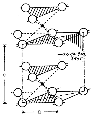
第1図 \text{CdI}_2 型結晶構造
