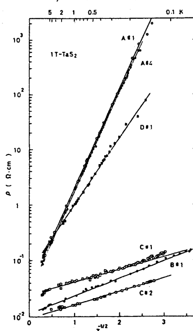
第7図 電気抵抗の T^{-1/2} 依存性
