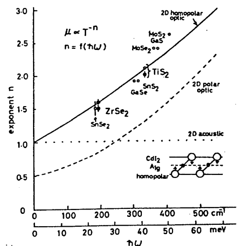
第4図 移動度 \mu の温度指数 n と光学同極フォノンのエネルギー \hbar\omega の関係を与えるFIVAZの図
