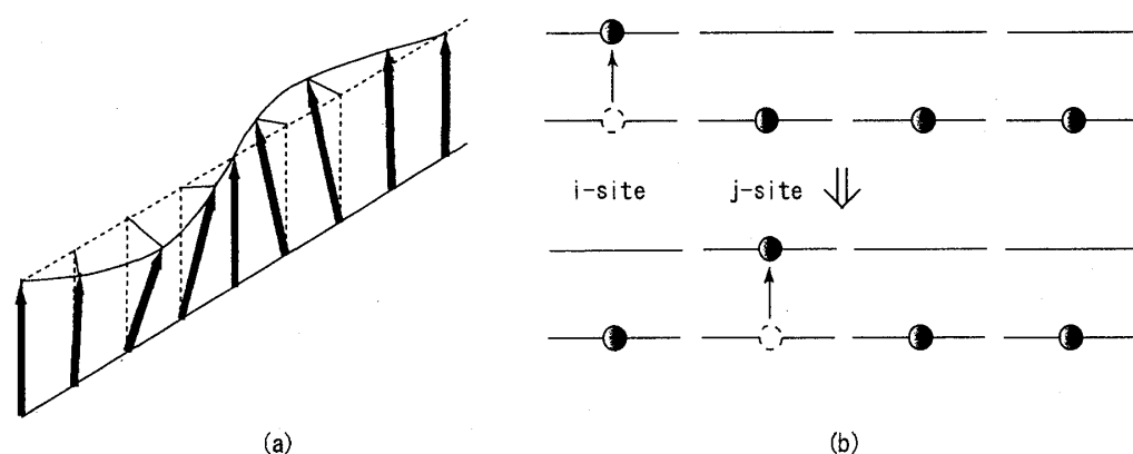
図 3: 磁気励起子媒介超伝導。(a) 磁気励起子の直感的イメージを与えるための図。ここでは強磁性をイメージして描かれているが、実際は反強磁性である。磁気励起子は、スピン波と同様、スピンの集団励起である。(b) 結晶場分裂した2準位系。 i サイトが励起状態から基底状態に落ち込むと、そのエネルギーは隣接する j サイトに伝えられ、それを励起する。これが、結晶全体に波として伝播するのが磁気励起子である。
