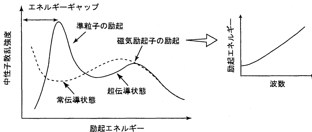
図 2: \text{UPd}_2\text{Al}_3 の中性子非弾性散乱スペクトルの模式図。超伝導の出現と同時に、エネルギーギャップが低エネルギー領域に現れる。高エネルギー側に見えるブロードなピークは磁気励起子の励起によるものであり、結晶を伝播する波であることを反映し、dispersion（右図のような波数依存）を示す。
