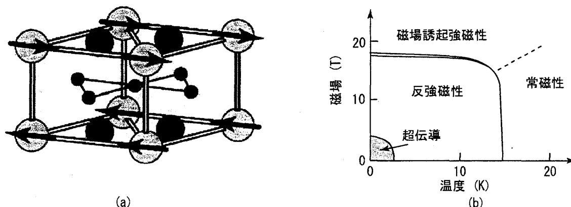
図1: UPd 2 Al 3 の結晶構造および磁気構造 (a) と磁場・温度相図 (b)。結晶構造は六方晶であり、ネール温度以下で生じる反強磁性秩序状態は、強磁性的な配列がc軸の方向に積層した構造となっている。反強磁性相内の低温領域で磁場を強くしていくと、18 T 付近でいわゆる「メタマグ」が生じる。これは磁化の飛びを伴う1次相転移であり、図(b)中の2重線の部分で観測される。常磁性状態でもメタマグの名残が見られ、その異常の起こる磁場・温度が破線で示されている。また、約2 K 以下で、反強磁性秩序を保ちながら、超伝導に転移する。
