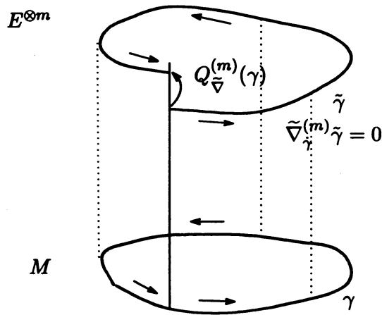
図 3: ホロノミー
