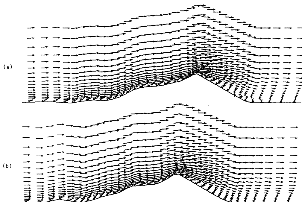
図4 一定時間経過後の砂丘形状と速度分布 (a)植生のない場合 (b)植生のある場合
