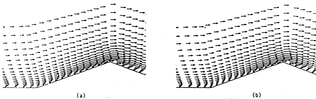
図3 初期の速度分布 (a)植生のない場合 (b)植生のある場合
