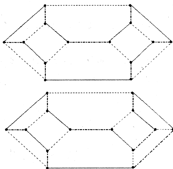
図 8 5-admissible でない例
