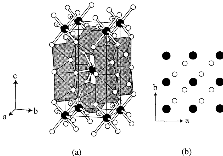
図 1: (a) トリルチル型化合物 \text{AB}_2\text{O}_6 の結晶構造。図中黒丸が A(遷移金属) 元素、白丸が酸素、灰色の多面体は \text{BO}_6 八面体を表す。(b) c 面の A 元素および酸素の配列
