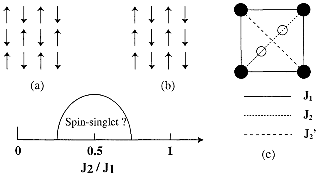
図 11: (a) 狭義の Néel オーダー、(b) collinear オーダー、および (c) c 面内における Cu 原子間の磁気相互作用の模式図
