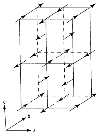
図 9: \text{CuSb}_2\text{O}_6 の磁気構造モデル
