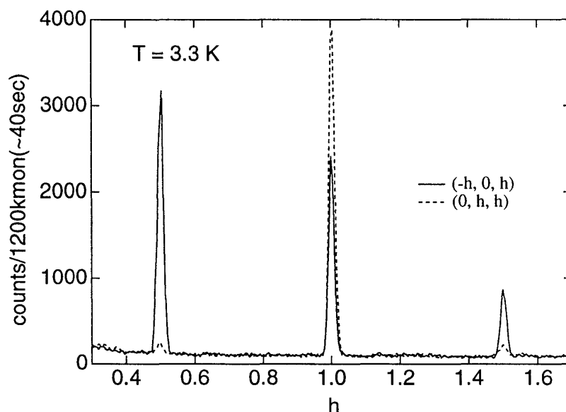
図 5: [-h,0,h]^* および [0,h,h]^* 方向への回折プロファイル
