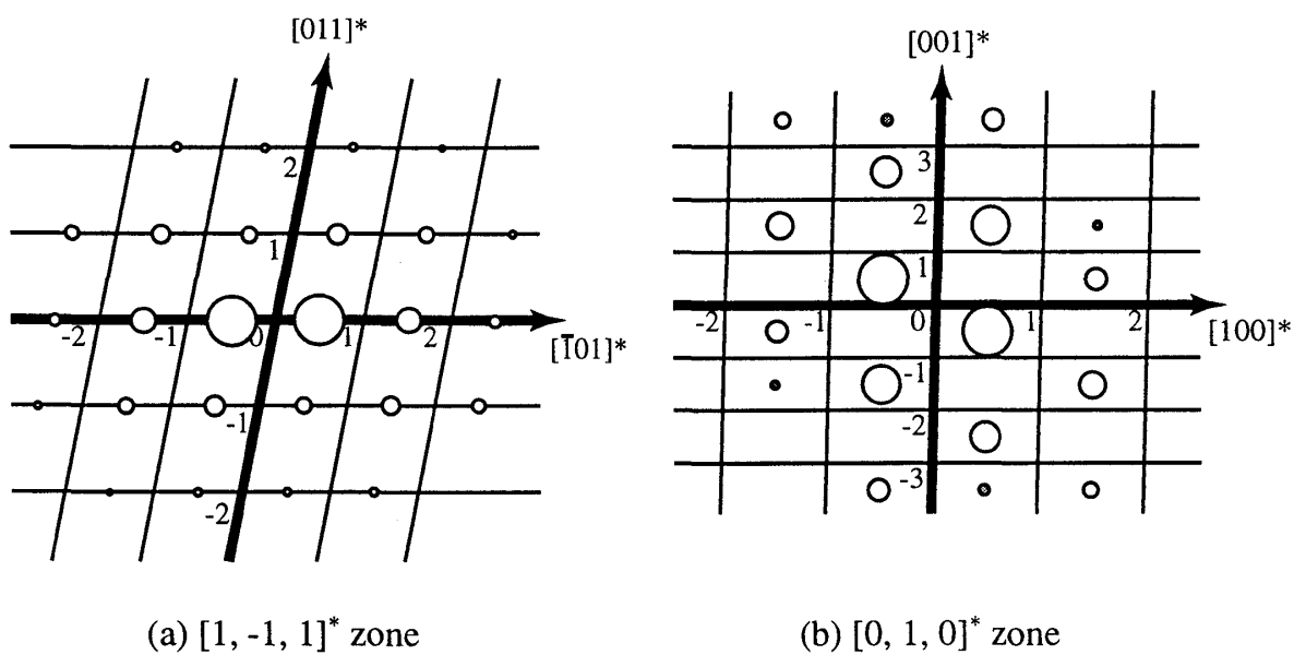
図 8: (a) [1, -1, 1]^* および (b) [0, 1, 0]^* ゾーンにおける各逆格子点で測定された反射強度。図中の円の面積が強度に比例する。磁気的な Bragg 反射のみ示してある。
