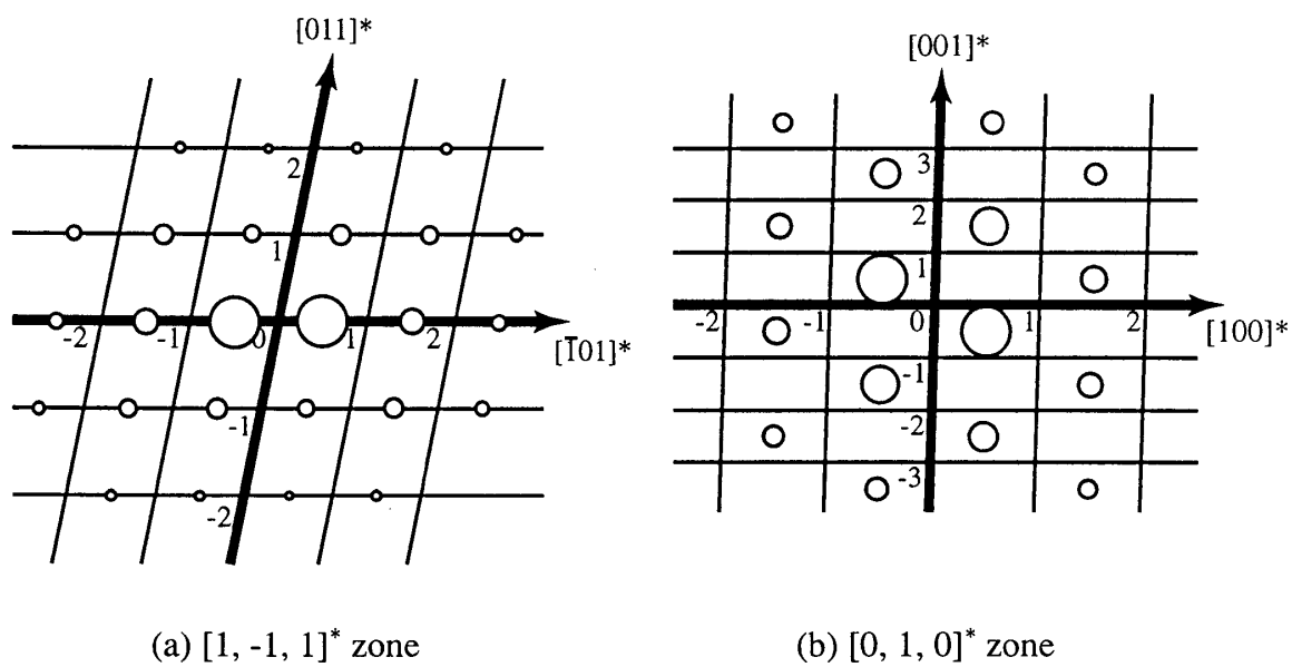
図 10: 磁気構造モデルからシミュレートした (a) [1, -1, 1]^* および (b) [0, 1, 0]^* ゾーンにおける回折強度
