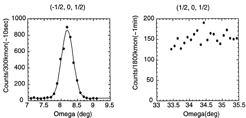
図 7: (-1/2, 0, 1/2) および (1/2, 0, 1/2) 反射の \omega スキャンプロファイル
