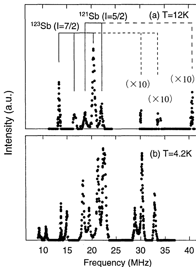
図 3: (a)12K および (b)4.2K においてゼロ磁場下で測定した周波数スペクトル
