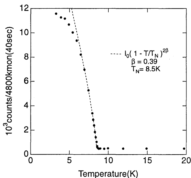
図 6: (-1/2, 0, 1/2) 反射強度の温度変化
