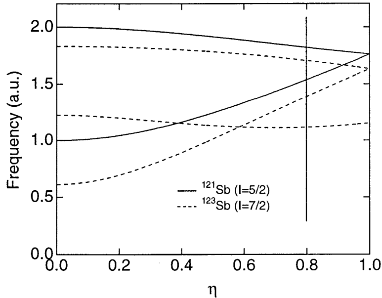
図 4: ^{121}\text{Sb} および ^{123}\text{Sb} 核の \nu_Q の \eta 依存性
