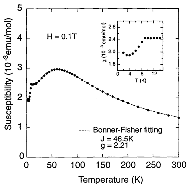
図 2: \text{CuSb}_2\text{O}_6 の帯磁率の温度依存性。内挿図は低温部を拡大したもの。
