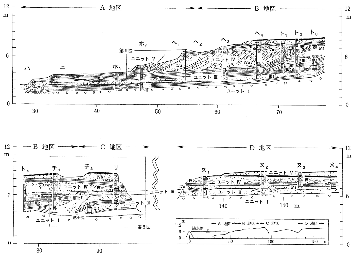
第6図 堆積様式を示す模式断面図。枠で囲った範囲の調査当時のスケッチと柱状図から作成したもの。チ 1 ～リのスケッチは第8図に、ホ 2 ～ヘ 1 については第9図に詳細を示す。
