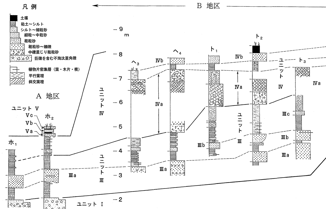
第7図 (その1) 各地点の柱状図 (おもにA～B地域)。高さは第5図に示した測量原点からの高さを表す。
