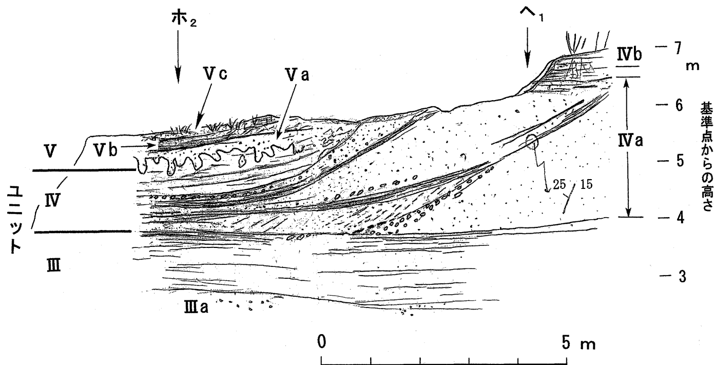
第9図 A地区東端部の堆積物のスケッチ。第6図ホ 2 〜ヘ 1 の範囲のスケッチで、筆者らのうちの中澤によるもの。
