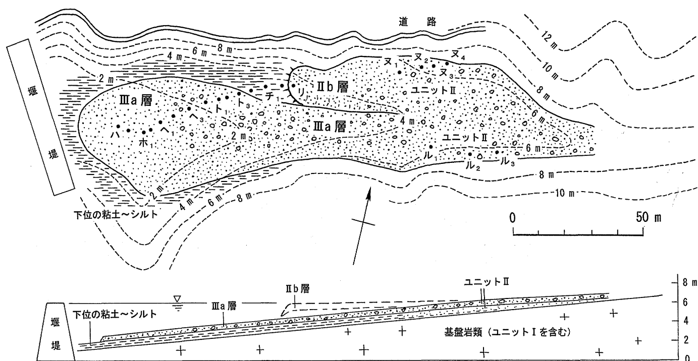
第10図 II bとIII a層の堆積過程復元図。等高線は堰堤建設直後の地形を復元したもの。6m等高線は本谷の池当初の水域を表す。
