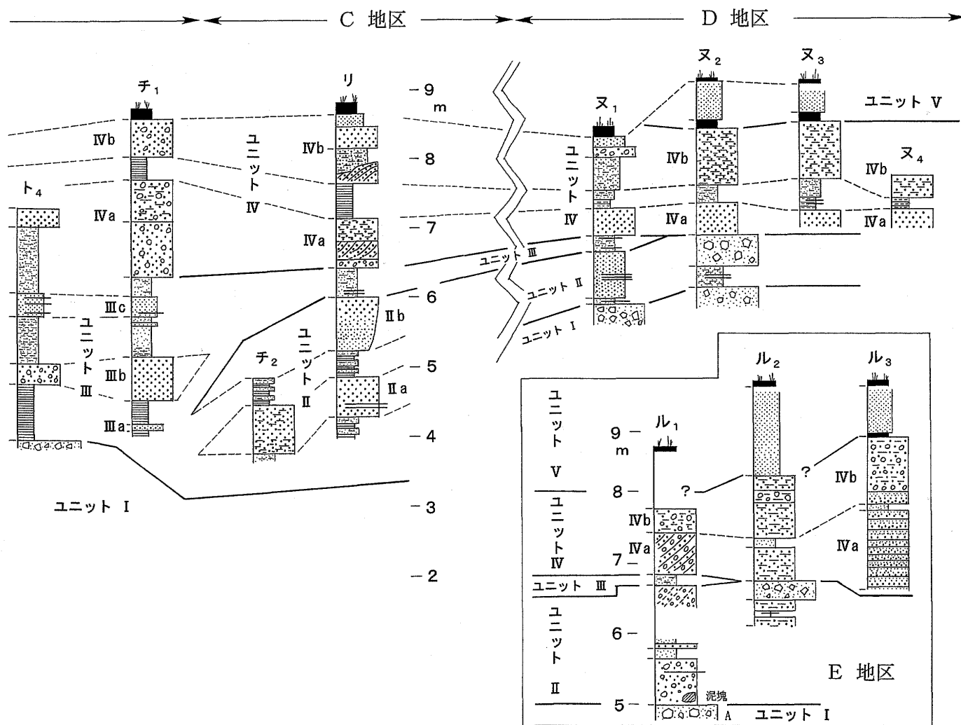
第7図 (その2) 各地点の柱状図 (おもにC～E地域)。説明はその1に同じ。
