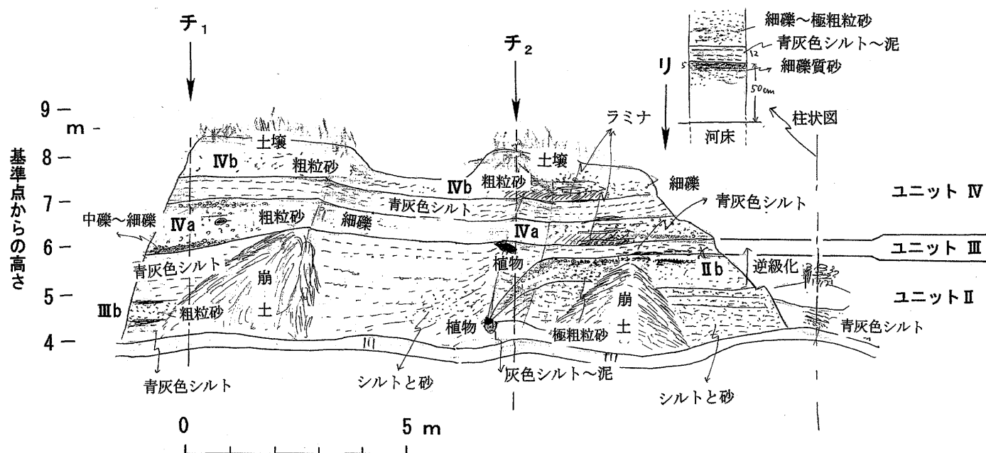
第8図 B地区東端〜C地区の堆積様式を示すスケッチ。第6図のチ 1 〜リ 1 の範囲のスケッチで、当時大学院生で調査に参加した故清水大吉郎氏によるもの。
