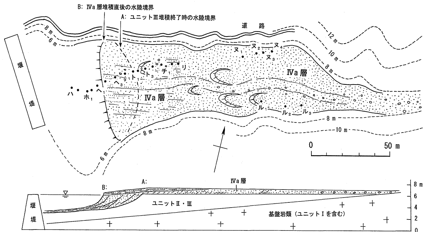
第 11 図 IVa 層の堆積過程復元図。破線はユニットⅢ堆積終了後の水陸境界，ハッチをつけた線はIVa 層堆積直後の水陸境界。
