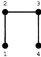
図 6: ネットワーク (N, L^5)
