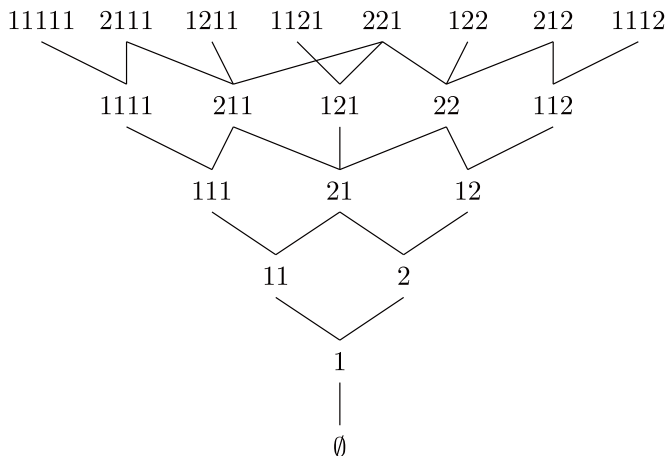
図 2: Young-Fibonacci 束の Hasse 図
