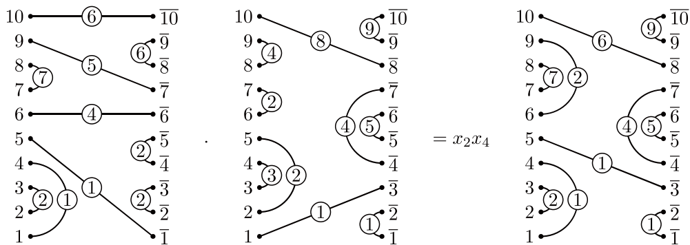
図 4: ラベル付き Temperley-Lieb 図式の積
