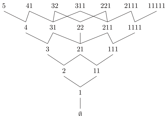
図 1: Young 束の Hasse 図
