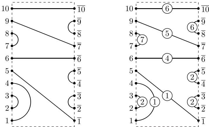
図 3: Temperley–Lieb 図式とラベルつき Temperley–Lieb 図式
