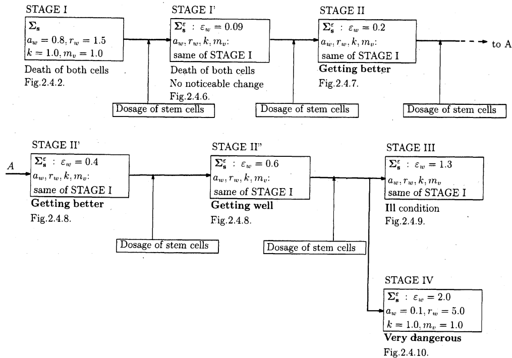
図 3.2: シミュレーションのシナリオとその結果：幹細胞の外部投与により幹細胞と成熟細胞がどのように増殖していくかをシミュレーションするためのシナリオ：STAGE I ではモデルを \Sigma_s とし幹細胞，成熟細胞共死滅するパラメータと設定する。この STAGE I に対して幹細胞の外部投与を行なう。したがって，STAGE I' 以降ではモデルは \Sigma_s^\varepsilon となる。まず，外部投与量 \varepsilon_w = 0.09 としたのが，STAGE I' であるが，外部投与量が少ないため改善は見られず両細胞とも死滅に至る。外部投与量 \varepsilon_w = 0.2 と増加させたのが，STAGE II である。この段階では両細胞とも死滅には至らないが，細胞数の収束値は両者ともごくわずかである。引き続き \varepsilon_w = 0.4, 0.6 と増加させるにしたがって両細胞の収束値は増えていくのが分かる (STAGE II', STAGE II'')。さらに \varepsilon_w = 1.3 と増加させると STAGE III の領域になり，細胞の癌化などのように無限に増殖し，両細胞共その数は発散してしまう。あるいは，モデルのパラメータを変えると STAGE IV のようになる場合がある。この場合の有意な平衡点は鞍点であるので，ここに収束するような初期値に設定するのは極めて困難であり危険な状態である。
