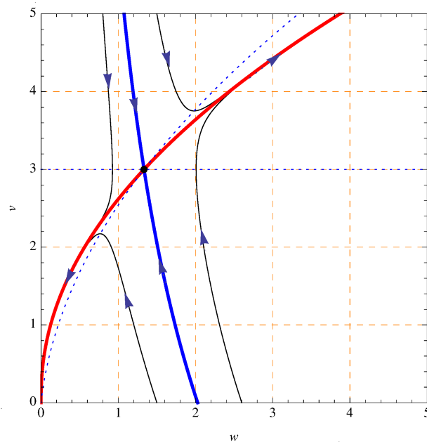
図 3.3: \Sigma_s^\varepsilon にて a_w = 0.1 , r_w = 5.0 , k = 1.0 , m_w = 1.0 とし, \varepsilon_w = 2.0 としたときの相図 (STAGE IV): 外部投与量が \varepsilon_w = 2.0 > 1 となり, R_w^\varepsilon < 1 となったため, 原点が沈点となり, 平衡点 E_1^\varepsilon が鞍点となった. その結果, 平衡点 E_1^\varepsilon に収束するような初期値に設定するのは極めて困難であり危険な状態と言える. すなわち, 特殊な場合の初期値を除いては両細胞共発散して細胞の癌化などが起こるか, あるいは, 両細胞共原点に収束し細胞死に至るかのどちらかである.
