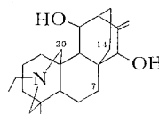
(418b) : C 20 -C 14 or C 20 -C 7
