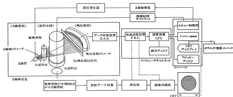
第1回 産業用、中エネルギー大線量X線CTスキャナ TOSCANER-3200 システムブロック。(撮影条件: 140KV, 300mA, スライス幅 0.5/2/5mm, スキャン領域 150/240/300mm \phi , スキャン速度 2.7/4.5/9 sec. CT画像: 画素寸法 0.3mm \times 0.3mm, マトリックス 320 \times 320, CT値 -1000 \sim 8000)。
