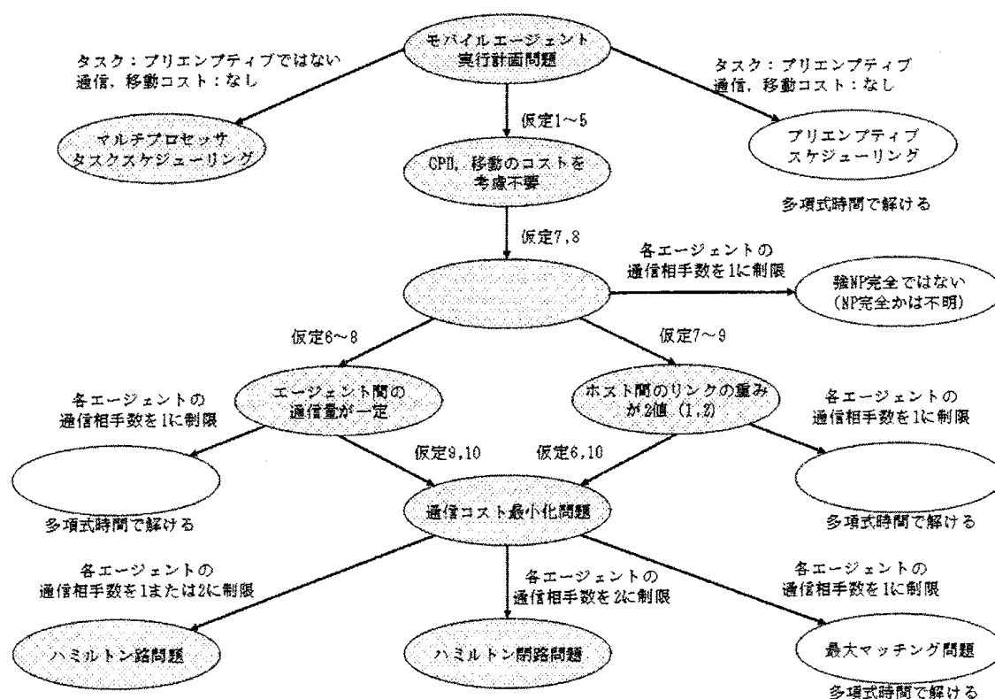
図 3: 問題の分類
