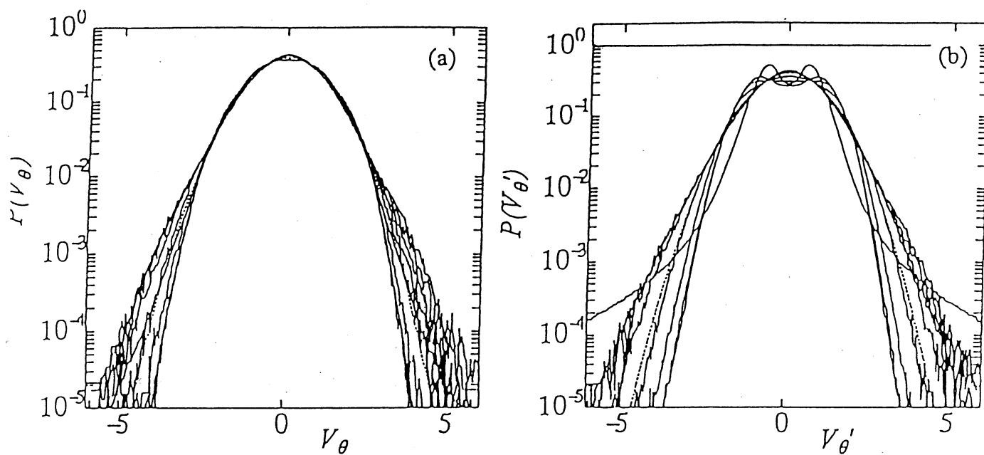
図1. スカラー相似変数のPDF。(a) 1次元サロゲートを用いなかった場合、(b) 1次元サロゲートを用いた場合。それぞれ、各実線が内側から r/\eta = 1.16, 2.32, 4.64, 9.38, \dots, 298 のようにスケールを大きくした時のPDFを示す。
