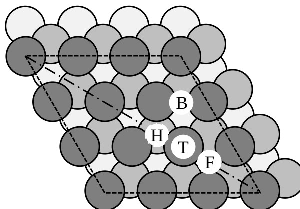
図 2 金 (111) 表面の吸着分子位置
