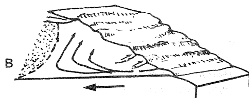
第1図 海洋底物質の上昇 COWAN (1978).
