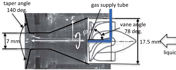
図 1: 旋回流型微細気泡発生器
