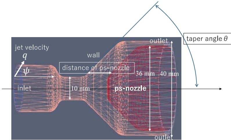
図 4: モデルノズル. inlet から流下方向に角度 \psi のジェットが生成, 生成された旋回流が圧力遮断ノズル:ps-nozzle 表面に沿ってノズル出口:outlet に至る. outlet では吸い込み流れはなく, ノイマン型の境界条件 or 流出条件を与える.
