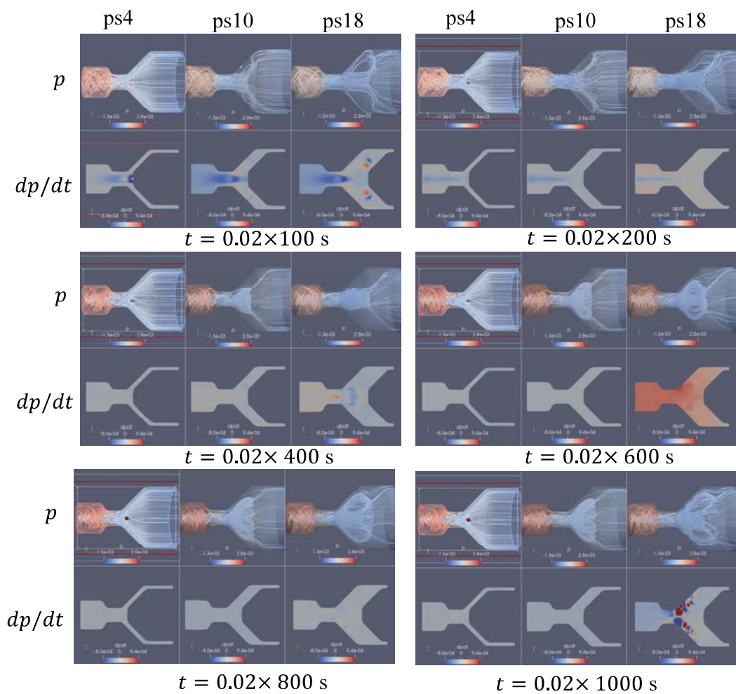
図 7: 圧力遮断ノズルの位置による渦崩壊過程. 図の上段は流線および流線上の圧力, 下段は軸対称面における圧力の時間変化率 dp/dt を示す. したがって, 定常状態の時, 下段の図は一律で 0 の色度を持つ.
