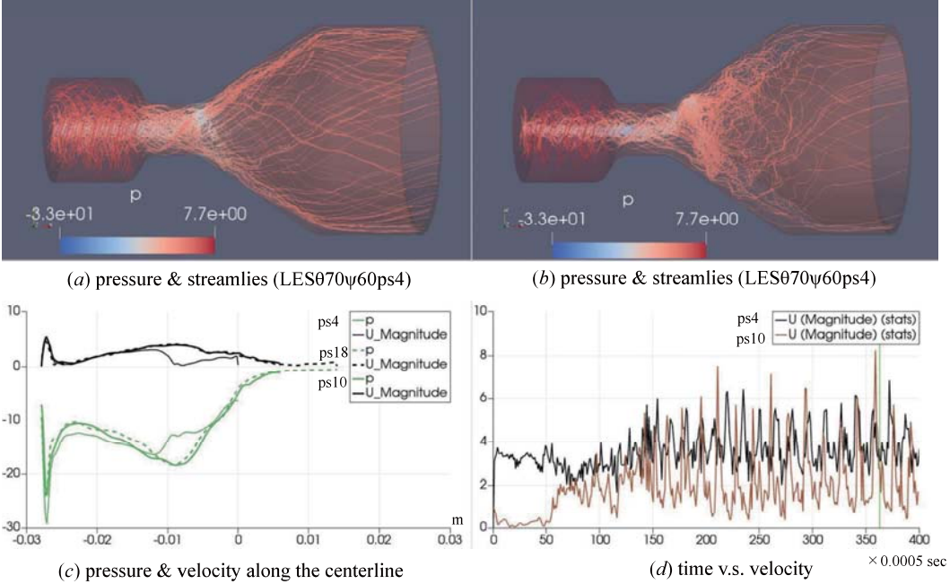
図 6: 圧力遮断ノズルの位置による (a),(b) 流況 (圧力および流線), (c) ノズル中心の圧力および流速, (d) テーパー部原点 ( x = 0, y = 0, z = 0 ) 近傍の圧力の時間変化. 図中 ps4, ps10, ps18 は, それぞれ d = 4, 10, 18 mmであることを示す.
