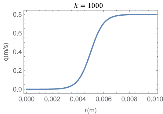
図 5: ベーンからの噴流: q(r) = q_0\{1 + \tanh k(r - R_v)\}/2 , q_0 = 0.8 \text{ m/s} , R_v = 0.01 \text{ m} for k = 1000 \text{ m}^{-1} . ここで, R_v は vane-swirler 砲弾部の半径である.
