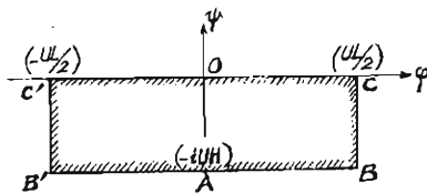
(b) W -plane
