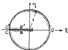
(c) \zeta -plane
