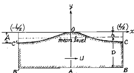
(a) z -plane
