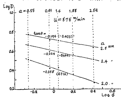
第4圖 紡糸孔板の厚さと纖維の直径
